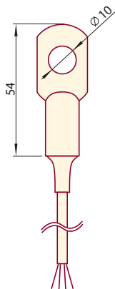
Рисунок 1. Внешний вид датчика
